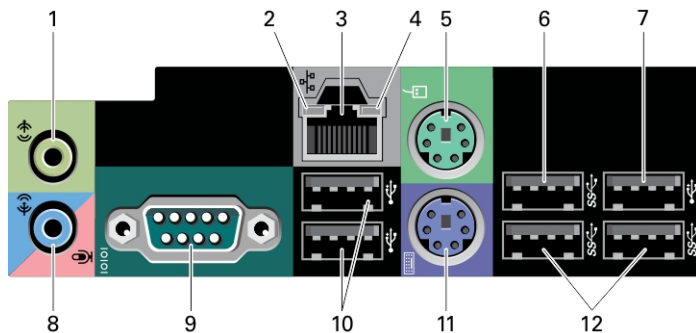
Obrázek 2. Pohled na zadní panel pracovní stanice T3610/T5610
