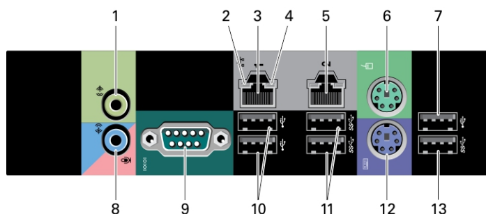
Obrázek 4. Zobrazení zadního panelu
