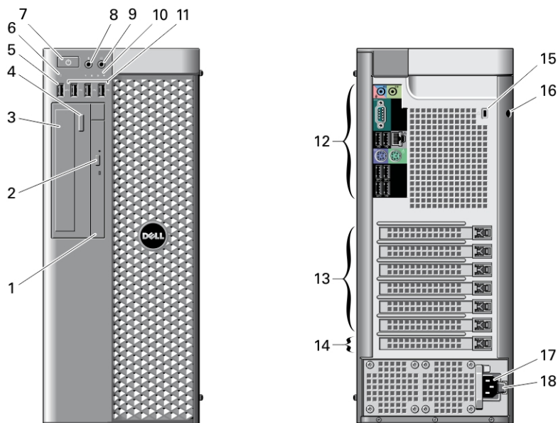
Obrázek 1. Čelní a zadní pohled na pracovní stanici T3610/T5610
