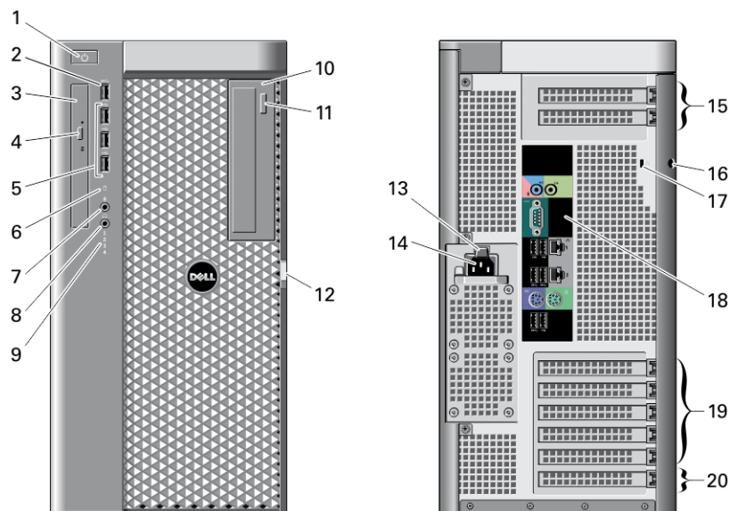
Obrázek 3. Čelní a zadní pohled na pracovní stanici T7610
